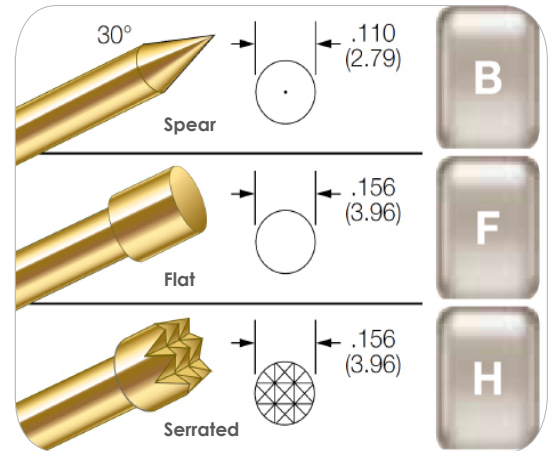
BKP-10 Pin Options
