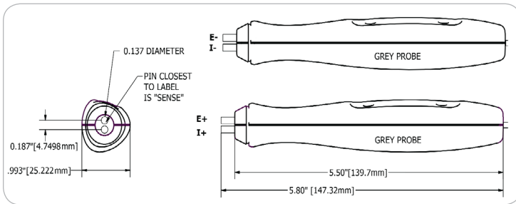
BKP-10 Probe Dimensions
